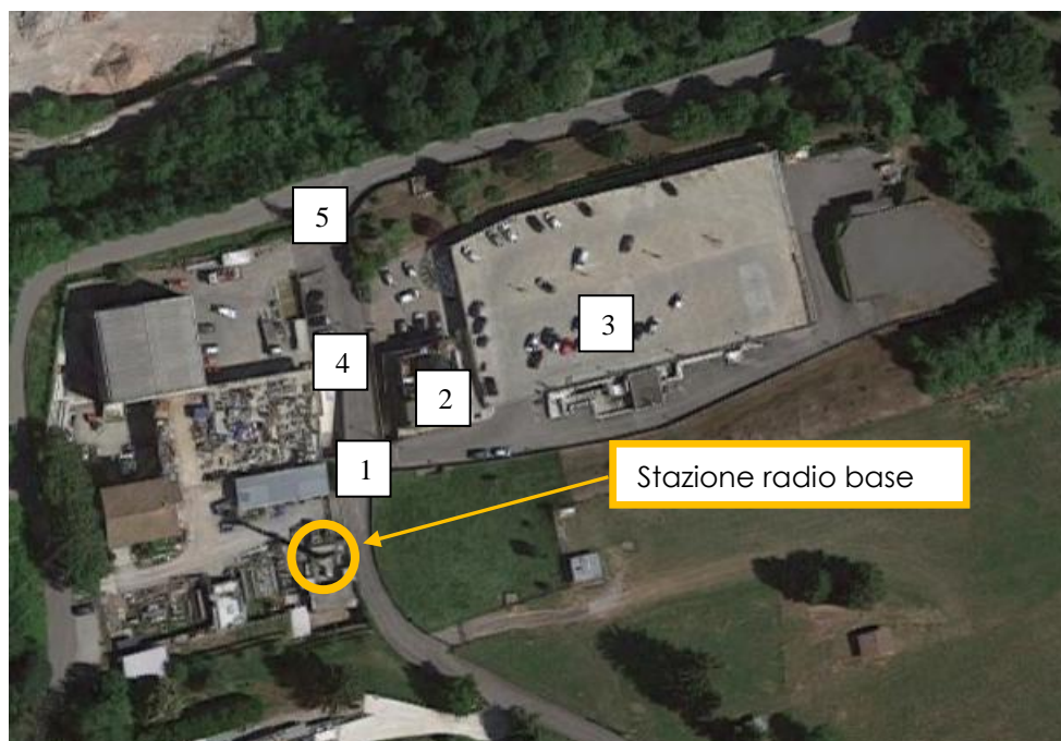
Figura 2: Ortofoto con indicazione degli impianti e dei punti di misura a banda larga
